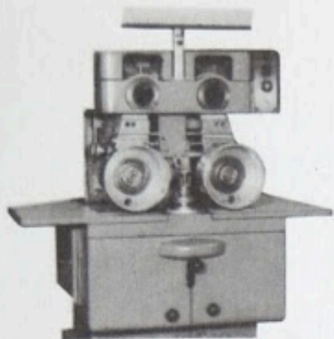
Полуавтомат Ф-328 для алмазной обработки наружных поверхностей часовых корпусов.
